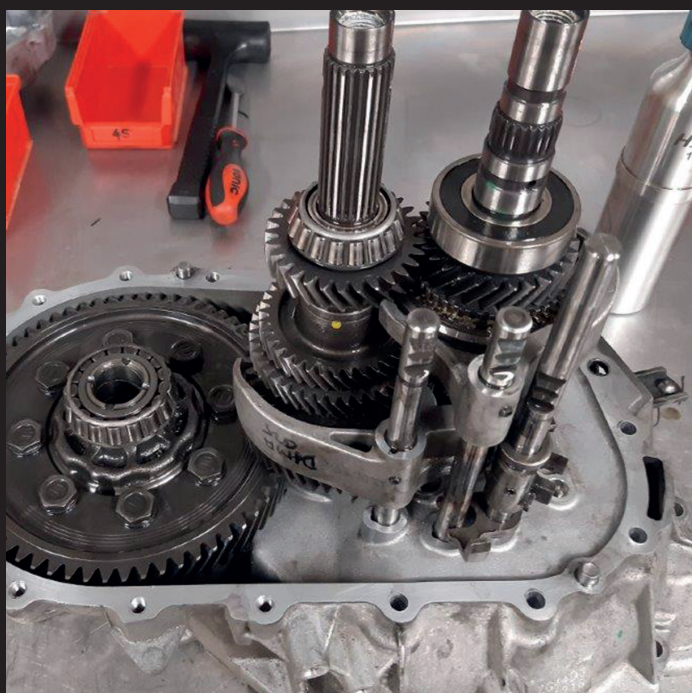
Getriebe-Revision
