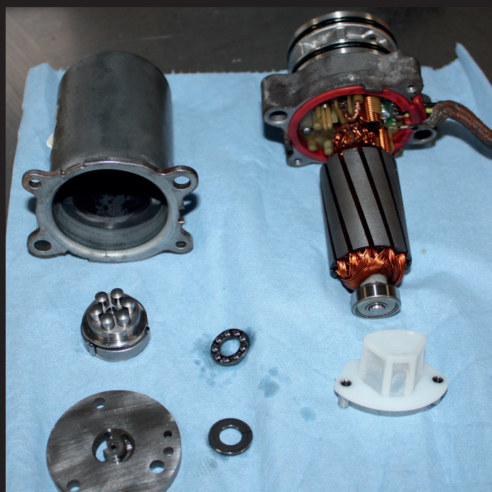
Haldexpumpe
